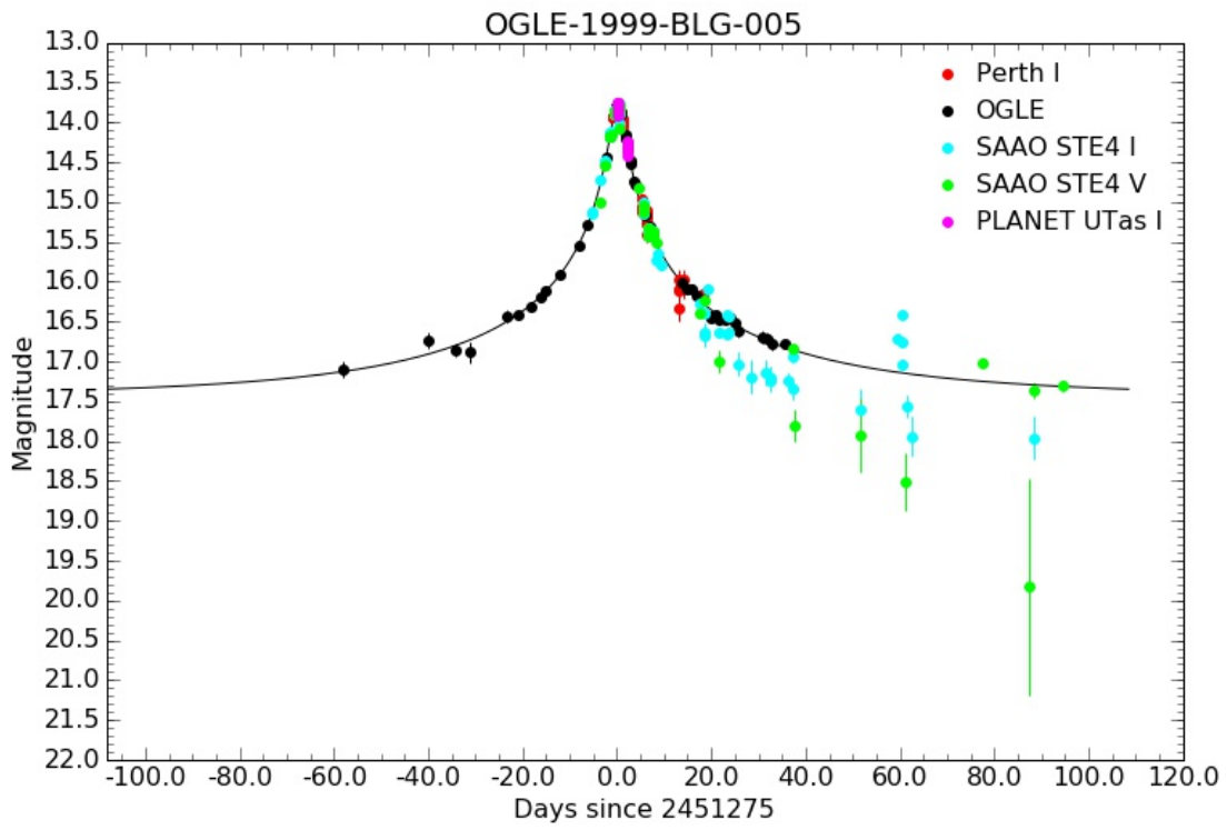
Fig. 12.— OGLE-1999-BLG-005
