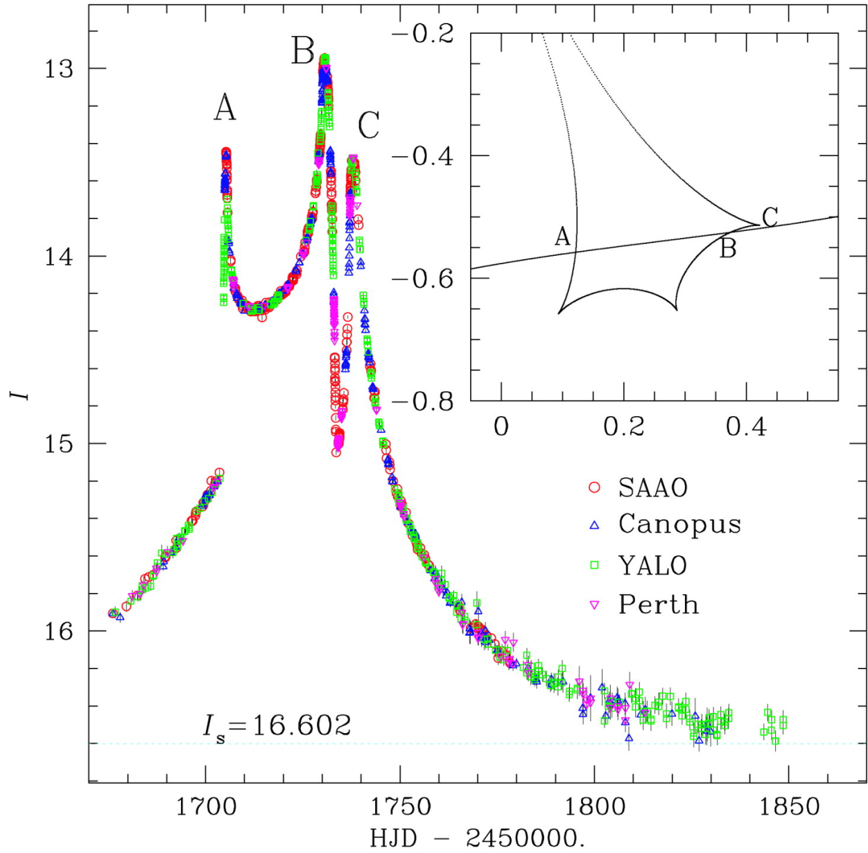
Fig. 19.— EROS-2000-BLG-005
