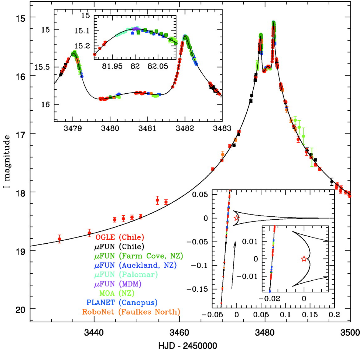
Fig. 17.— OGLE-2005-BLG-071
