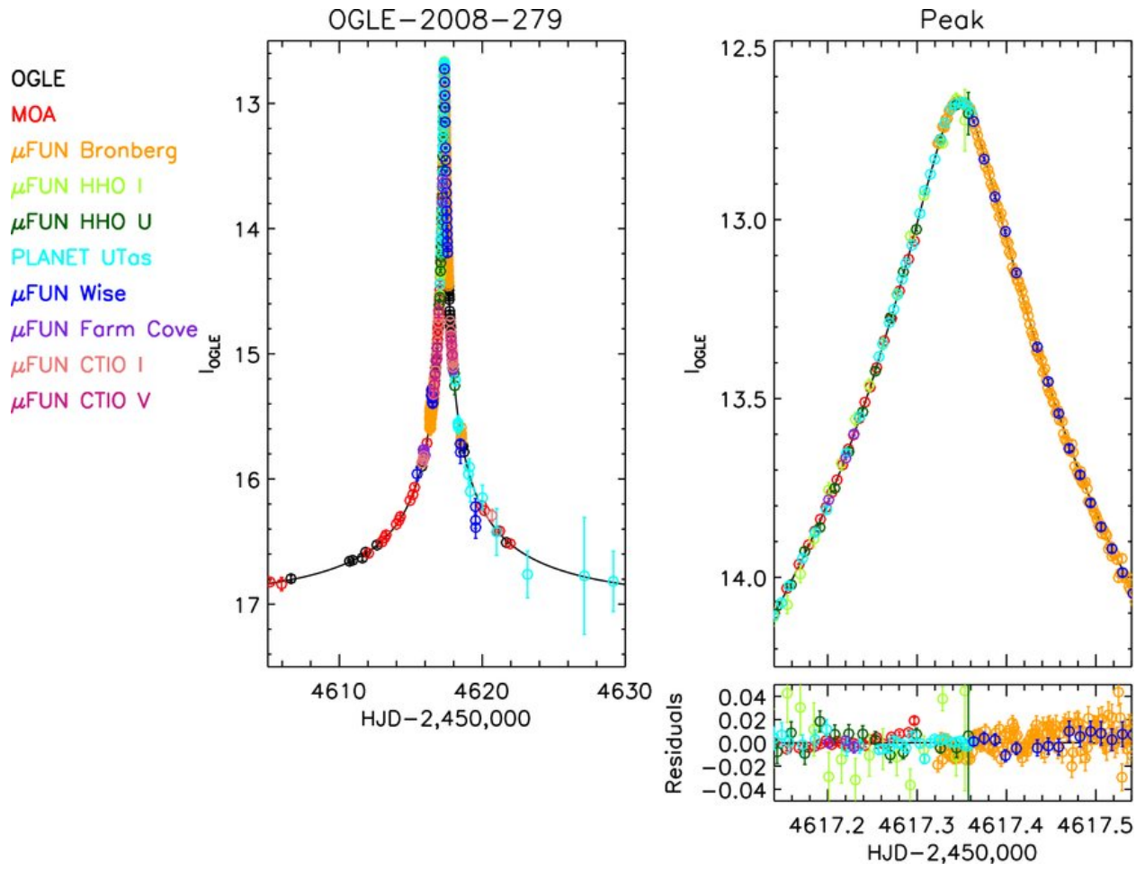
Fig. 13.— OGLE-2008-BLG-279
