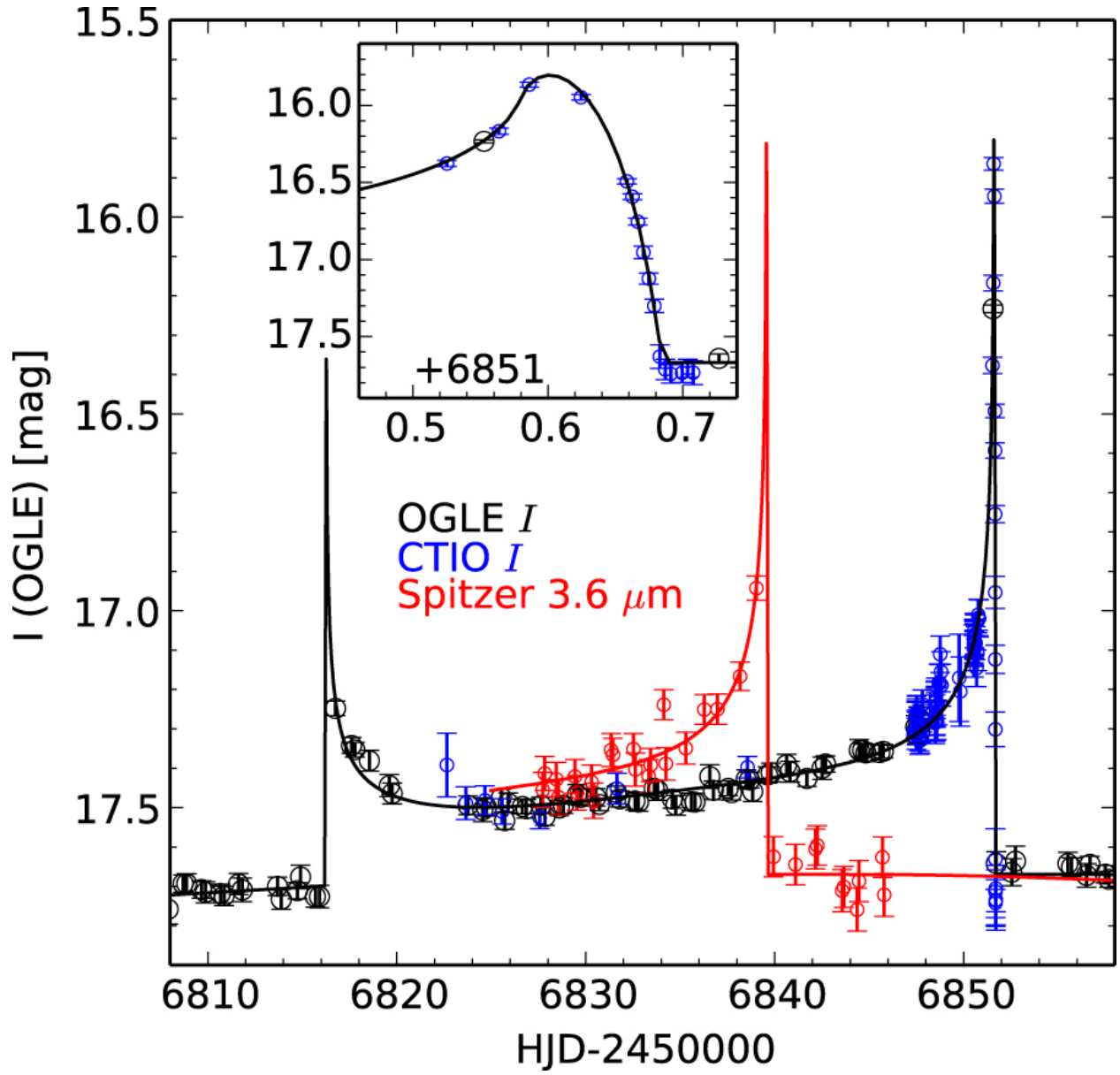
Fig. 5.— OGLE-2014-BLG-1050
