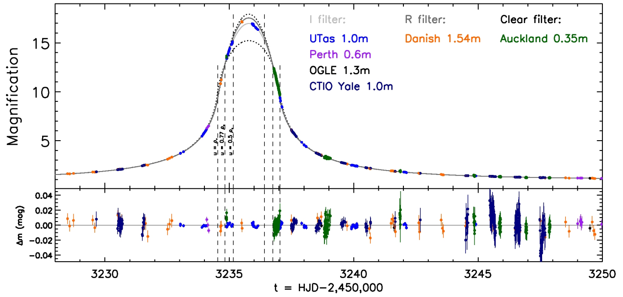
Fig. 6.— OGLE-2004-BLG-482
