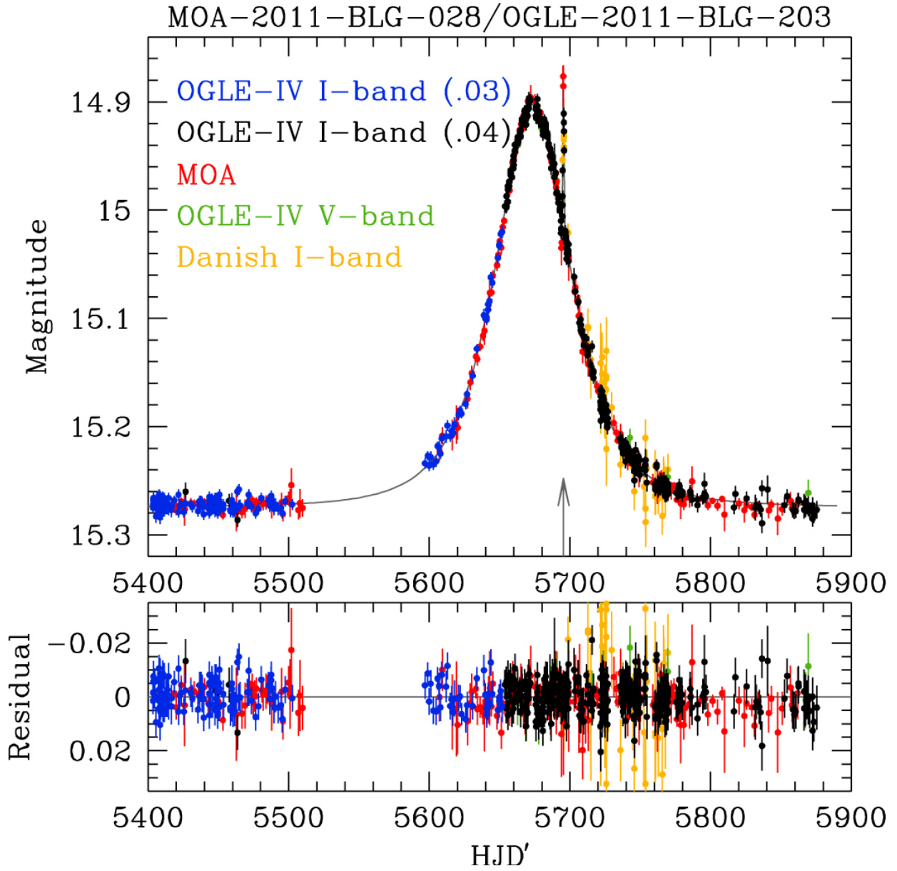
Fig. 18.— MOA-2011-BLG-028
