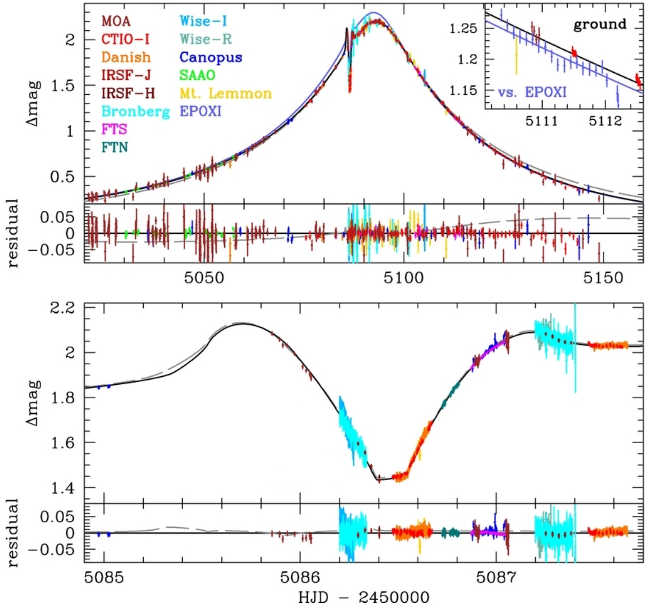
Fig. 10.— MOA-2009-BLG-266
