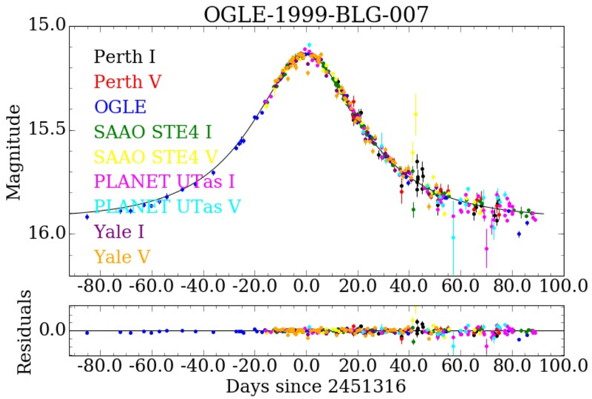
Fig. 20.— OGLE-1999-BLG-007
