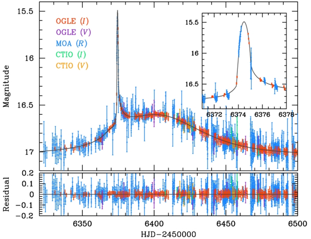
Fig. 16.— OGLE-2013-BLG-0102
