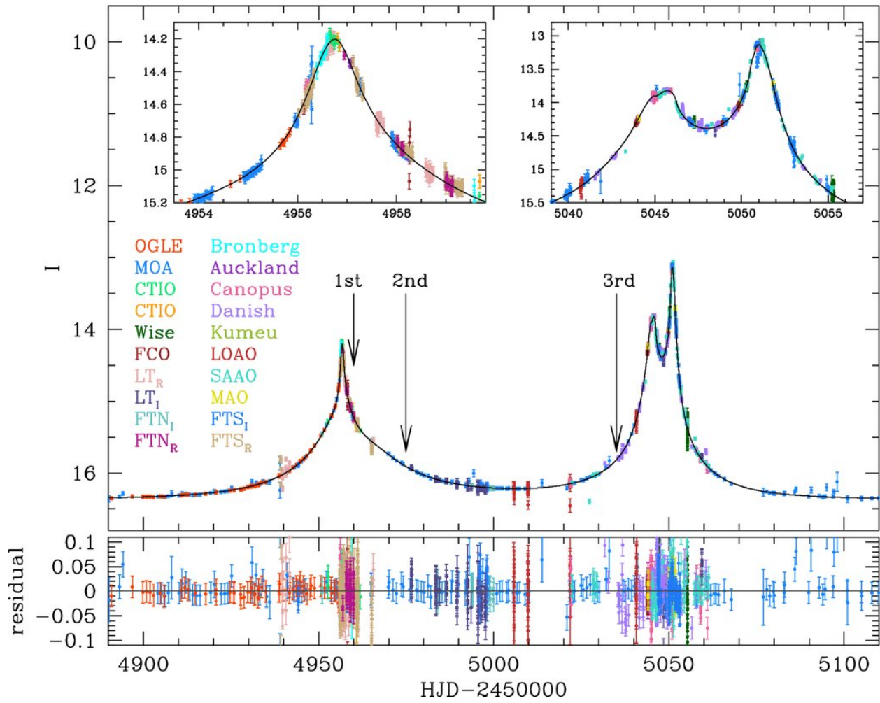
Fig. 8.— OGLE-2009-BLG-092
