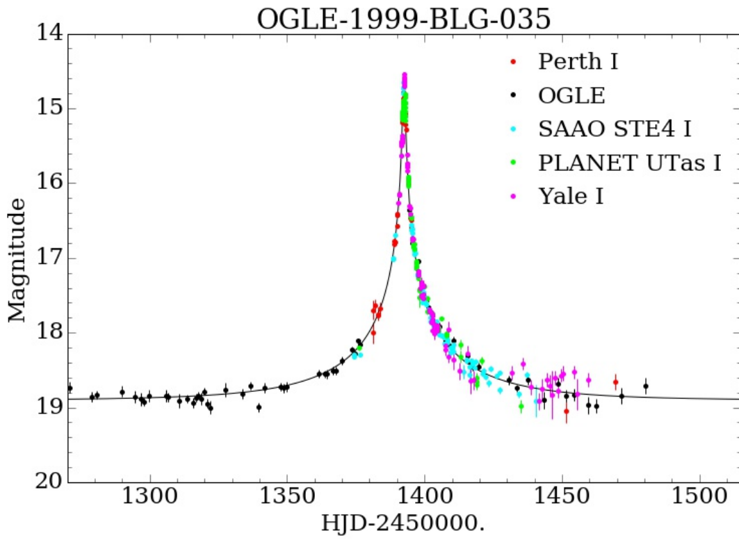
Fig. 4.— OGLE-1999-BLG-035
