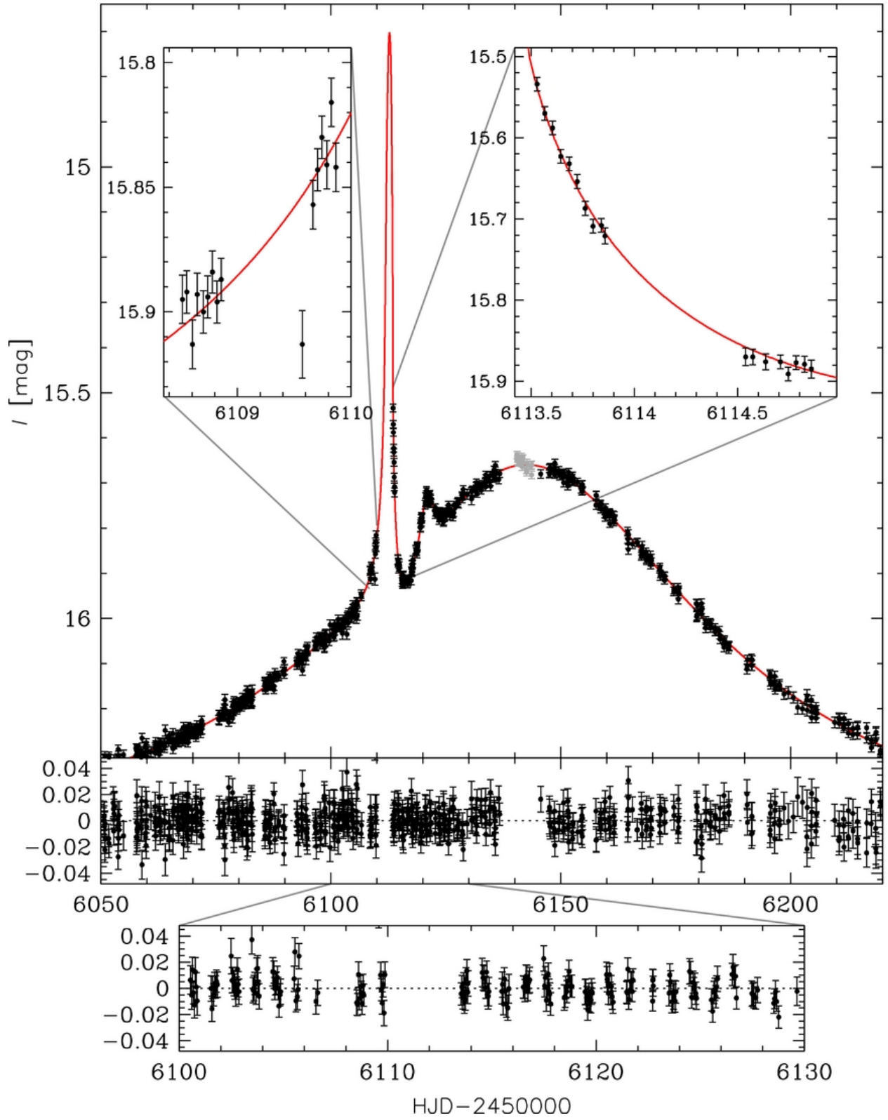
Fig. 2.— OGLE-2012-BLG-0406
