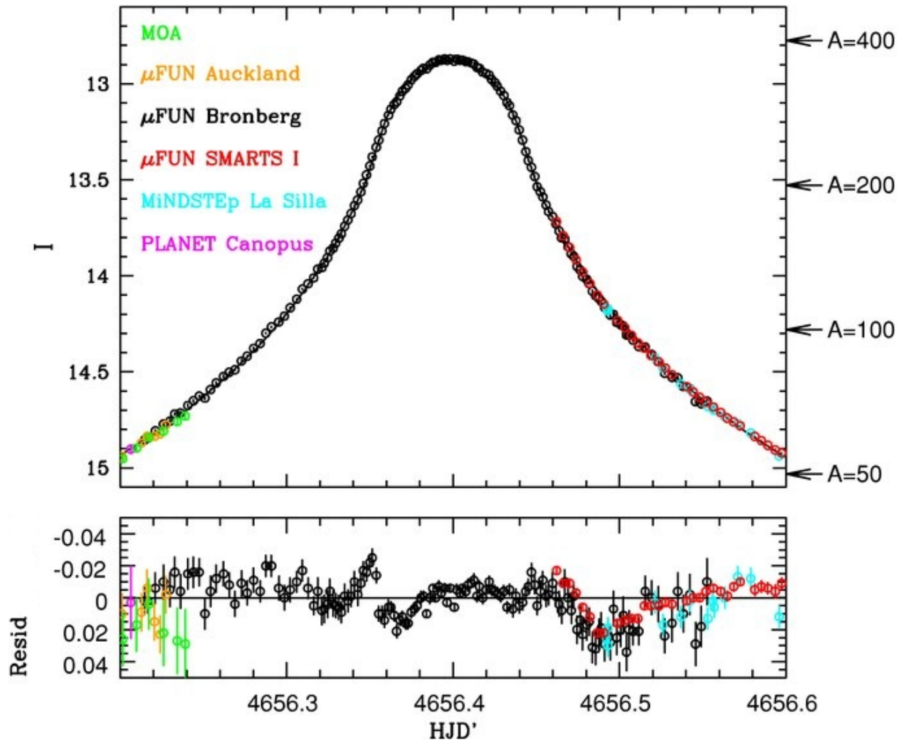
Fig. 15.— MOA-2008-BLG-310
