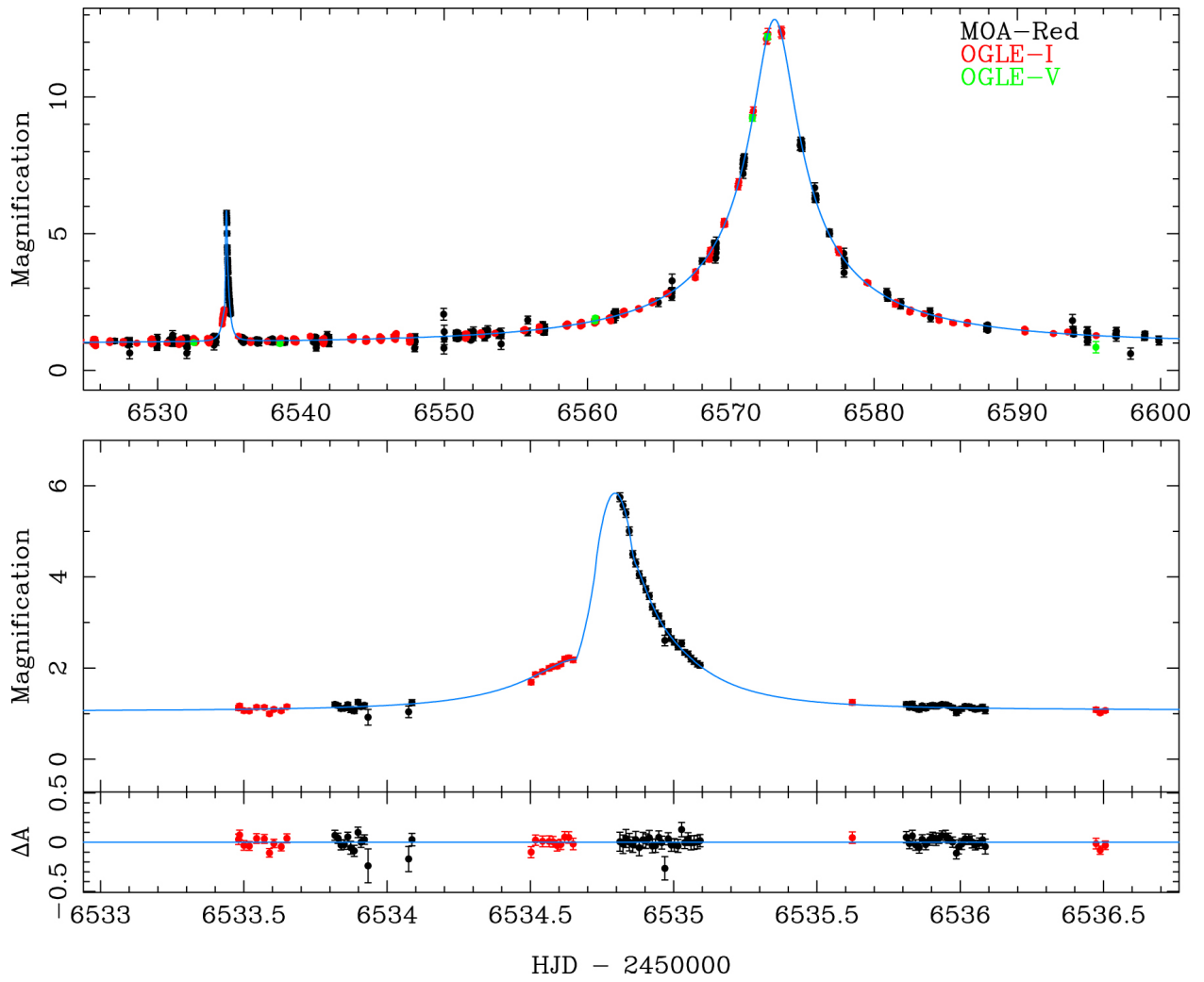
Fig. 1.— MOA-2013-BLG-605
