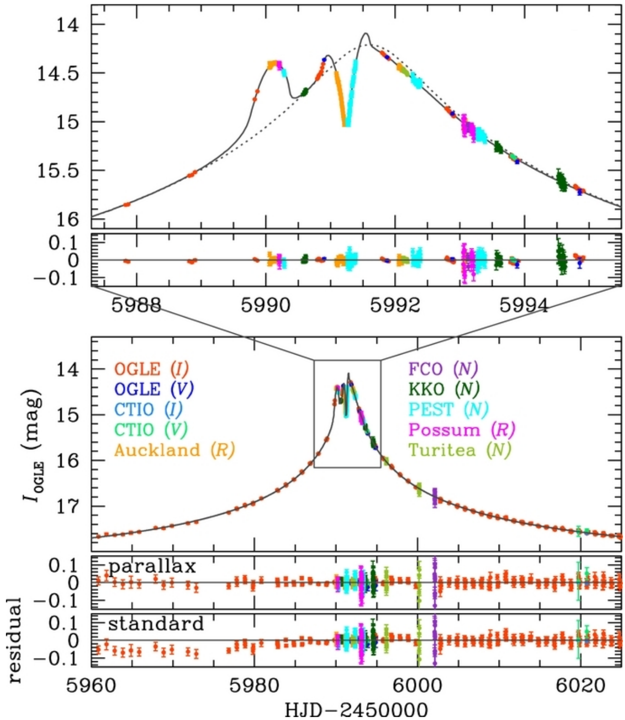
Fig. 7.— OGLE-2012-BLG-0026
