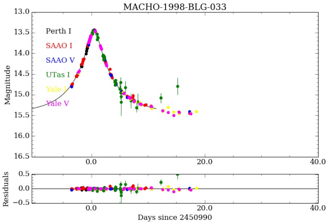
Fig. 11.— MACHO-1998-BLG-033
