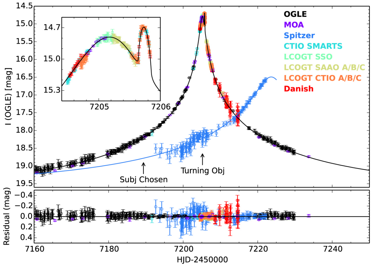
Fig. 3.— OGLE-2015-BLG-0966
