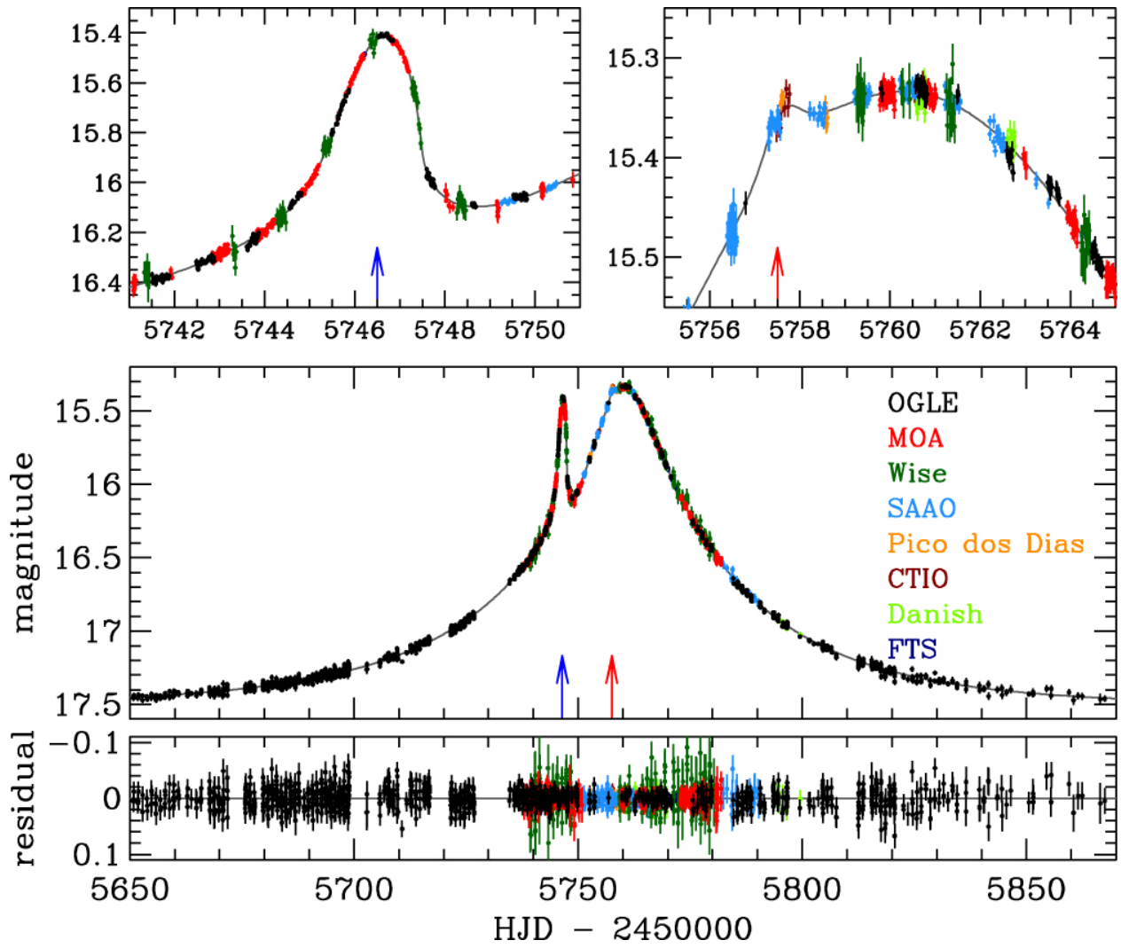
Fig. 8.— OGLE-2011-BLG-0265
