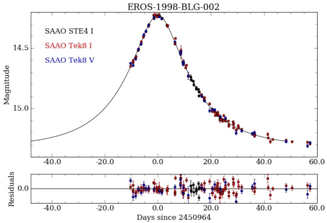
Fig. 10.— EROS-1998-BLG-002
