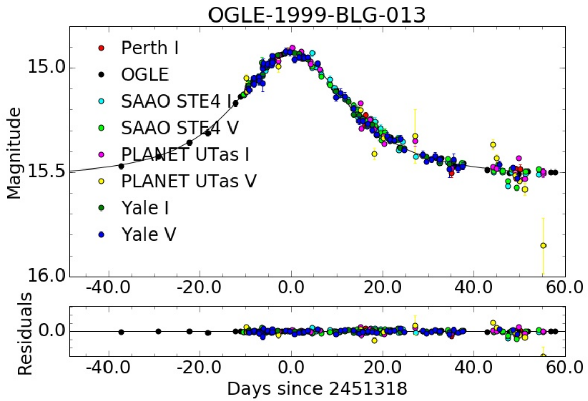
Fig. 4.— OGLE-1999-BLG-013
