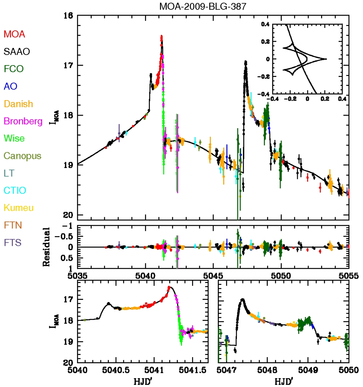
Fig. 2.— MOA-2009-BLG-387
