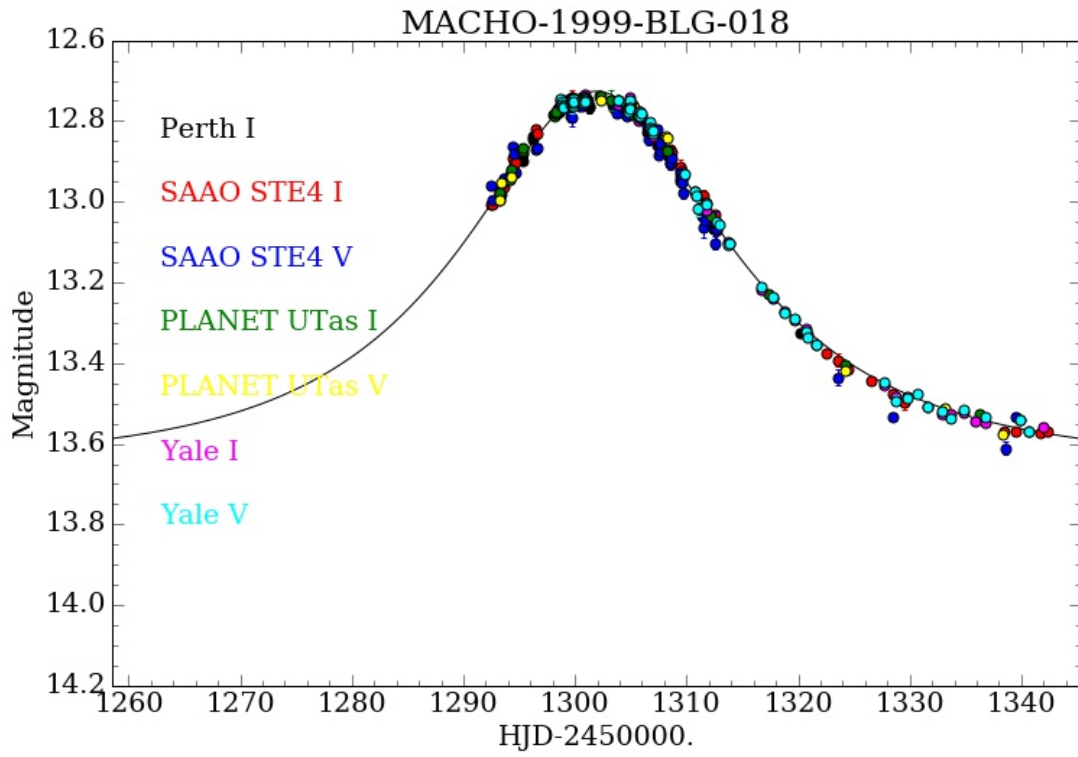
Fig. 3.— MACHO-1999-BLG-018
