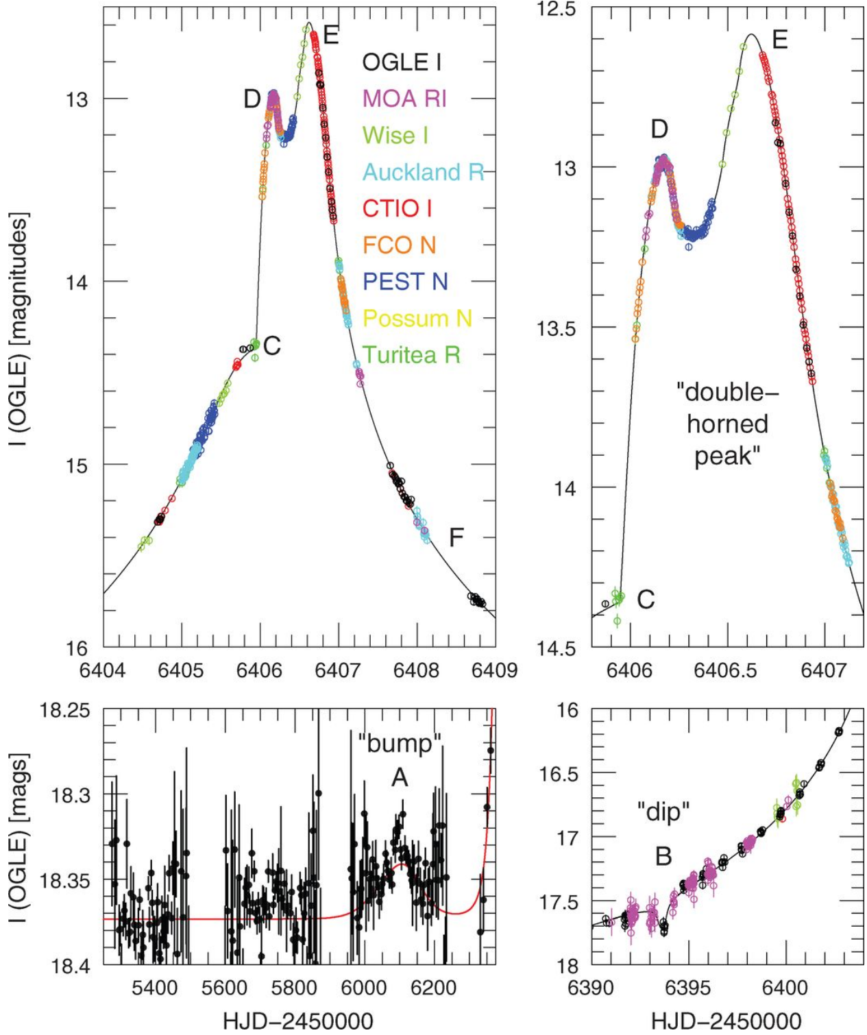
Fig. 9.— OGLE-2013-BLG-0341
